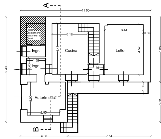
PIANTA PIANO PRIMO - Scala 1/100 -
